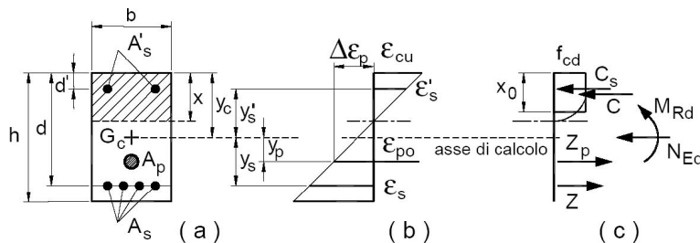
Fig. 4.1.4 – Sezione pressoinflessa
