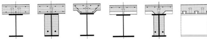
Fig. 4.3.3 -Tipologie di sezione composte per travi
