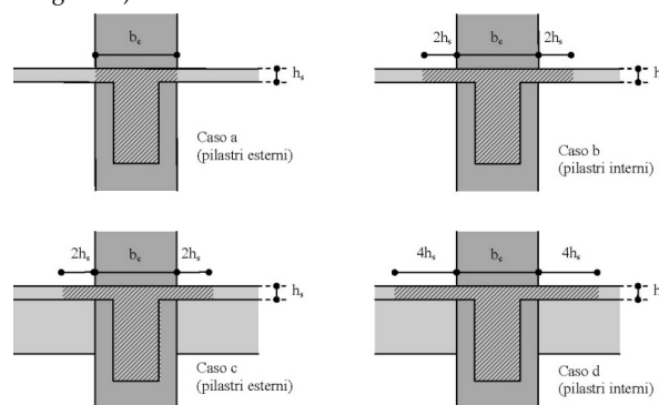
Fig. 7.4.1 – Larghezza collaborante delle travi
