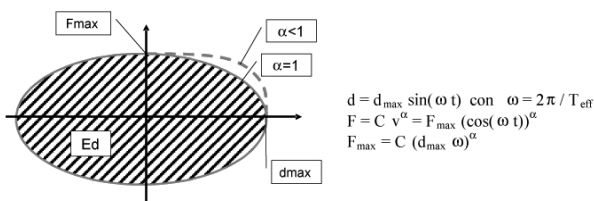
Fig. 11.9.2 – Dispositivi a comportamento viscoso
