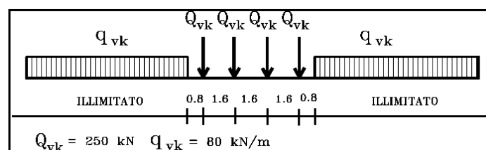
Fig. 5.2.1 - Modello di carico LM71
