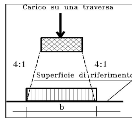
Fig. 5.2.4 - Distribuzione longitudinale dei carichi attraverso il ballast
