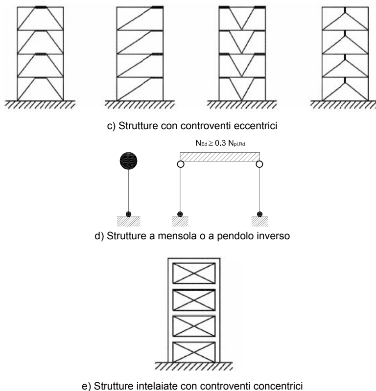
Fig. 7.5.1. - Tipologie strutturali
