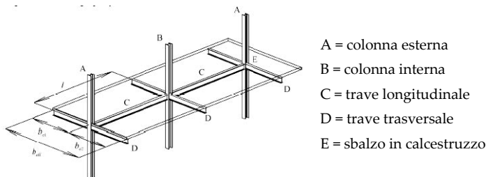
Fig. 7.6.2 - Definizione degli elementi in una struttura intelaiata
