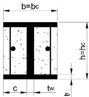
Fig. 7.6.1 - Rapporti dimensionali
