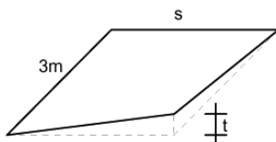
Fig. 5.2.14 - Sghembo ammissibile
